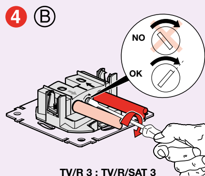
TV/R 3 ; TV/R/SAT 3
